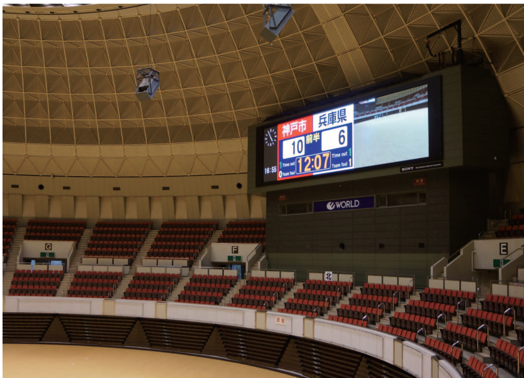
ワールド記念ホールに設置された大型LEDビジョン。主にホール内で開催されるバスケットボールやバレーボール、フットサルやテニス等のスポーツ競技大会で、得点板、時刻表示等として使用している。サイズは、W14,336mm×H4,096mm(587inch)。
